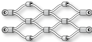
Randausbildung H24
